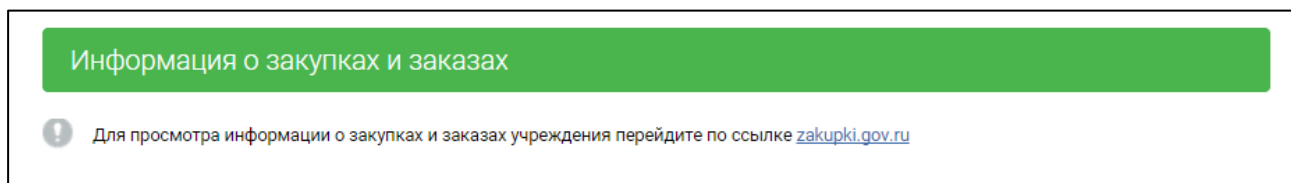
Рисунок 99. Информационное сообщение
