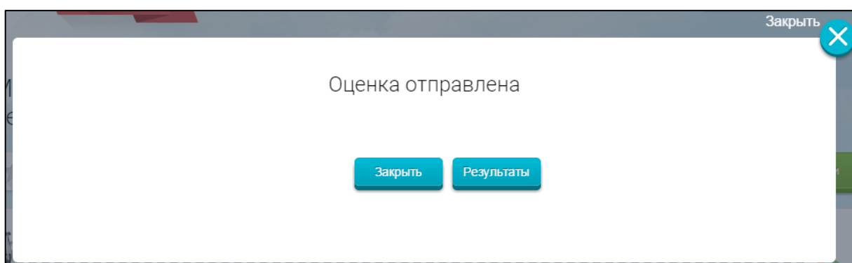
Рисунок 68. Информационное сообщение
