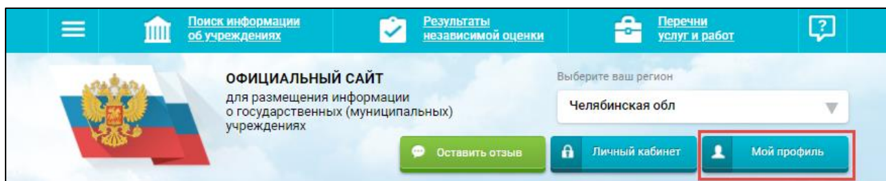
Рисунок 304. Создание профиля
