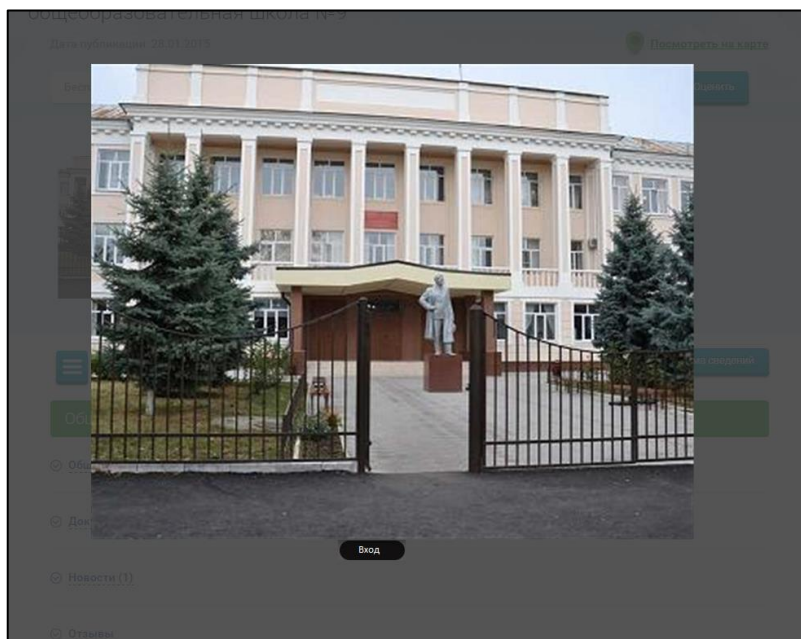
Рисунок 97. Отображение изображения
